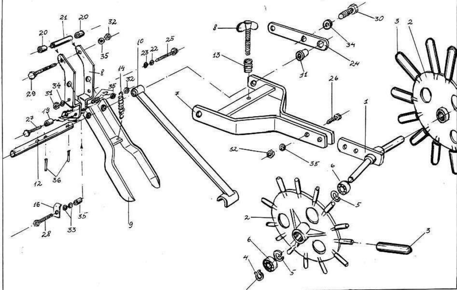
Аппарат высевальной (задняя часть)
