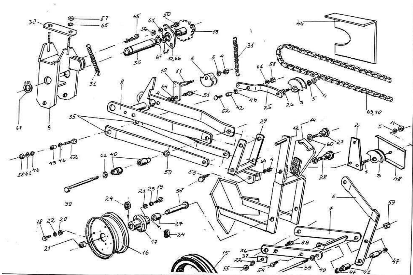
Аппарат высевальной (передняя часть)
