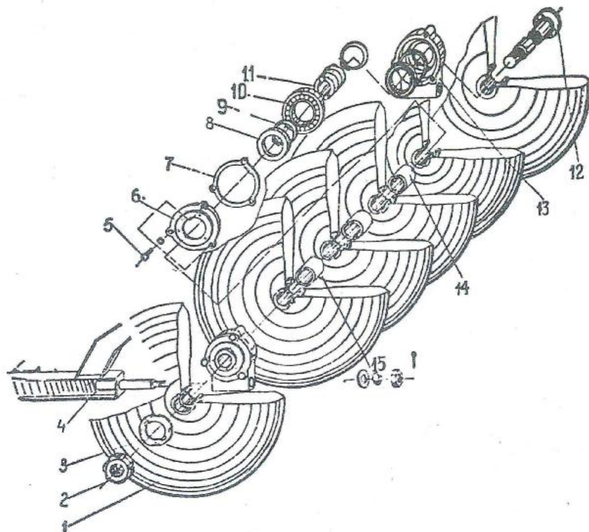
Рис. 22 Средняя секция прикатывающих катков СЗЮ 00.070
