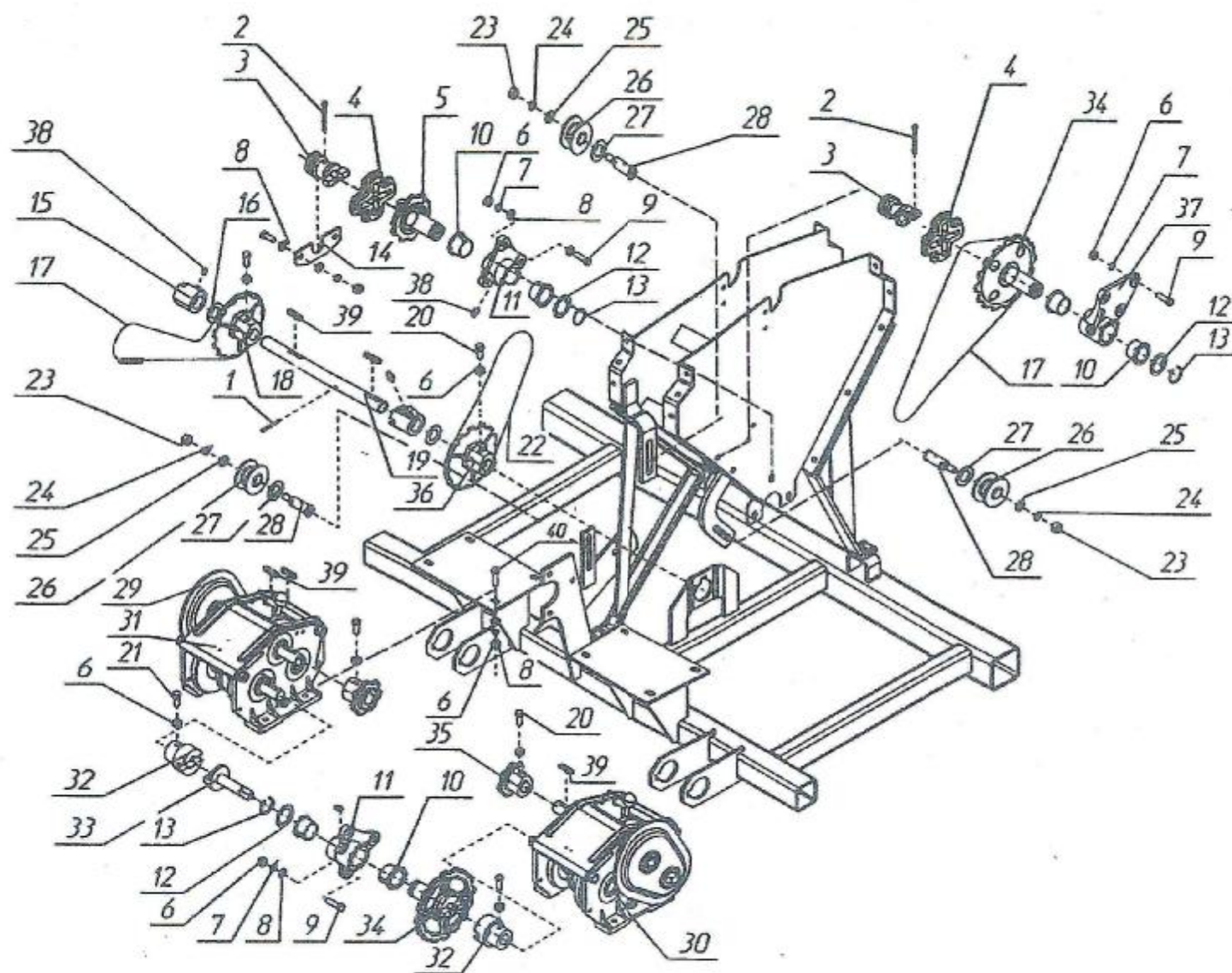
Рис. 18 Механизм привода зерновых и туковых высевальных аппаратов
