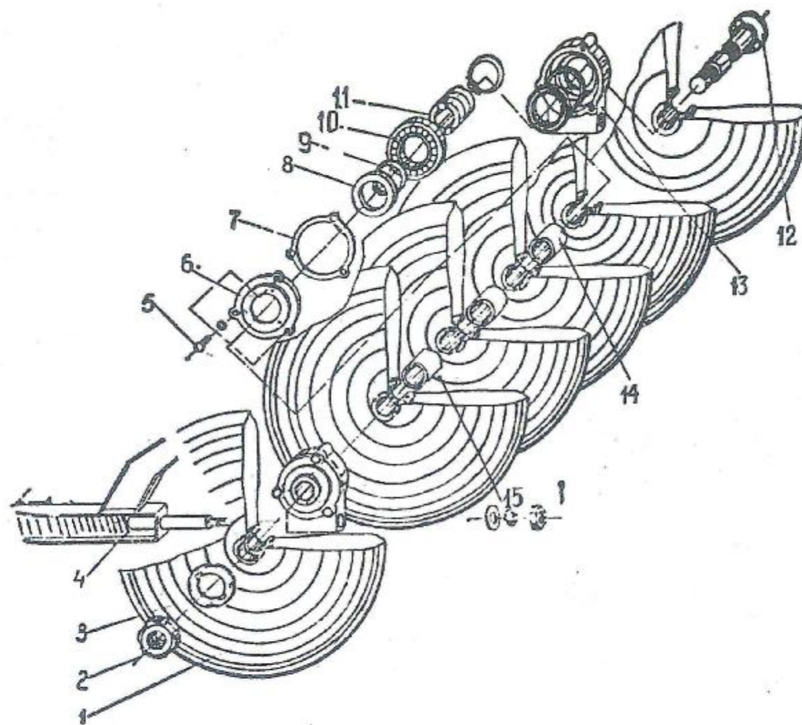
Рис. 24 Правая секция прикатывающих катков СЗЮ 00.090А
