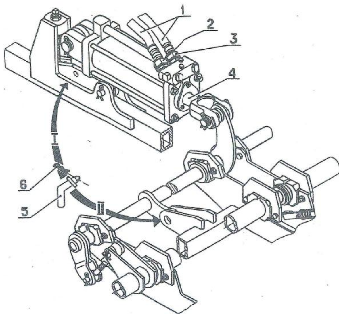
Рис. 8 Установка гидроцилиндра
