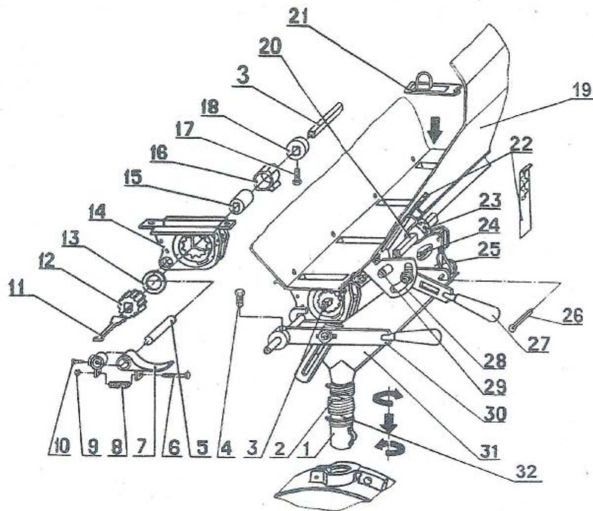
Рис. 14 Зерновой и туковый высевальные аппараты
