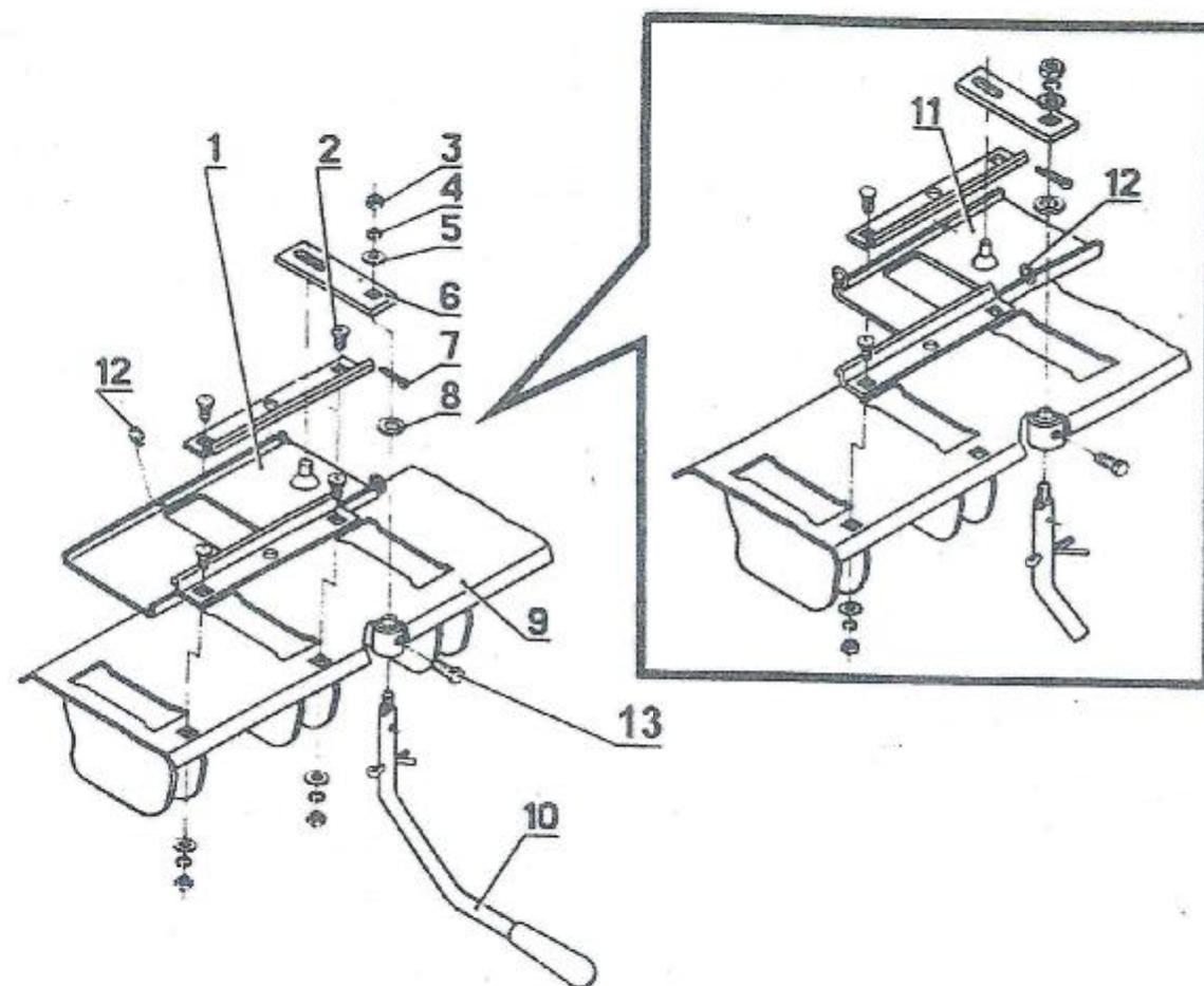
Рис. 16 Устройство для перекрытия зерновых аппаратов
