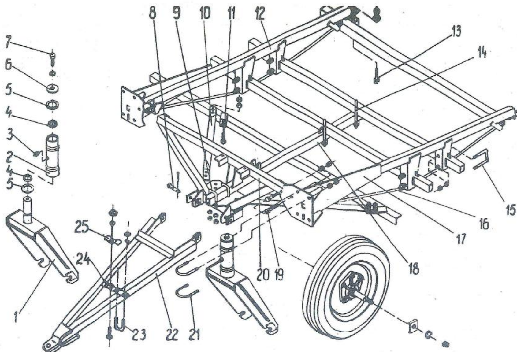
Рис. 5 Установка прицепа, сниц и колес с вилками
