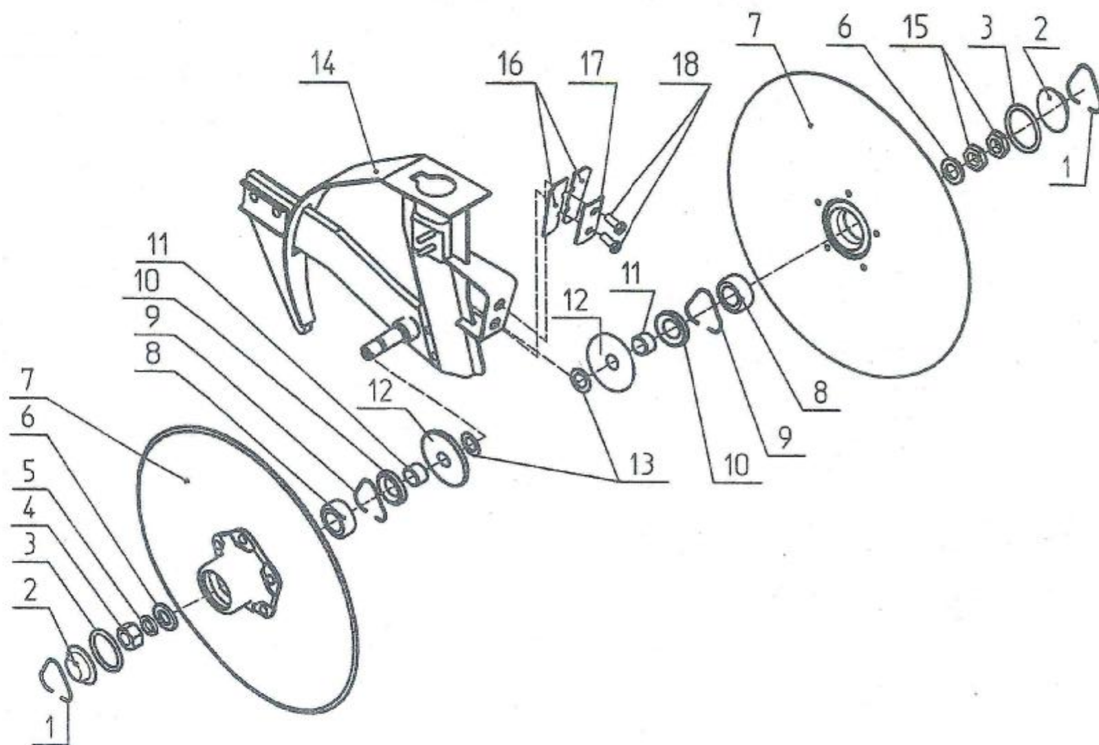
Рис. 11 Сошник 108.00.2580-06
