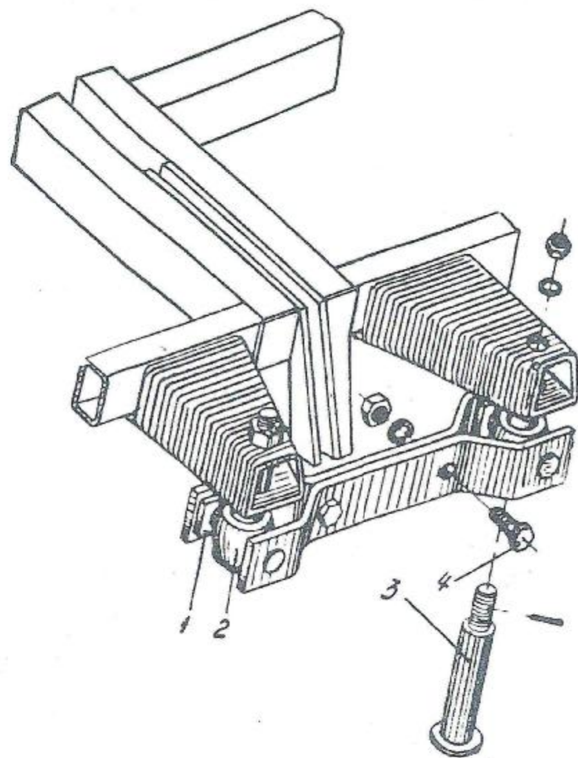
Рис. 28 Соединение смежных сеялок в агрегат
