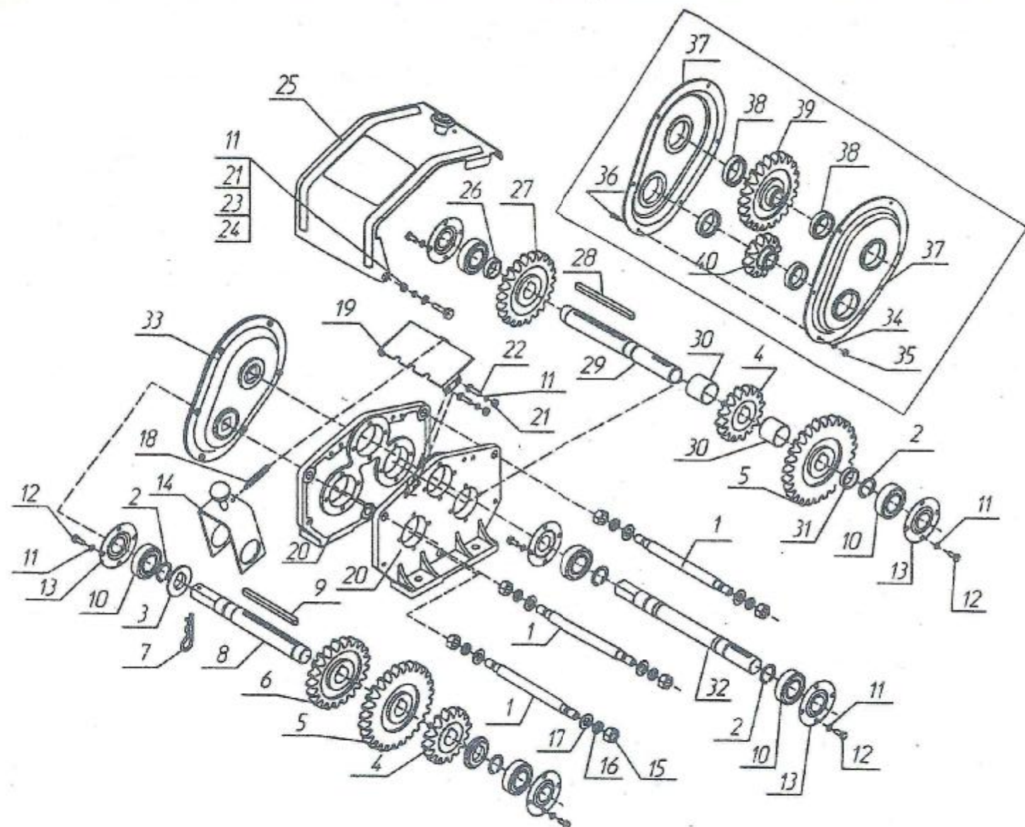
Рис. 20 Механизм передач 108.00.2020А-03
