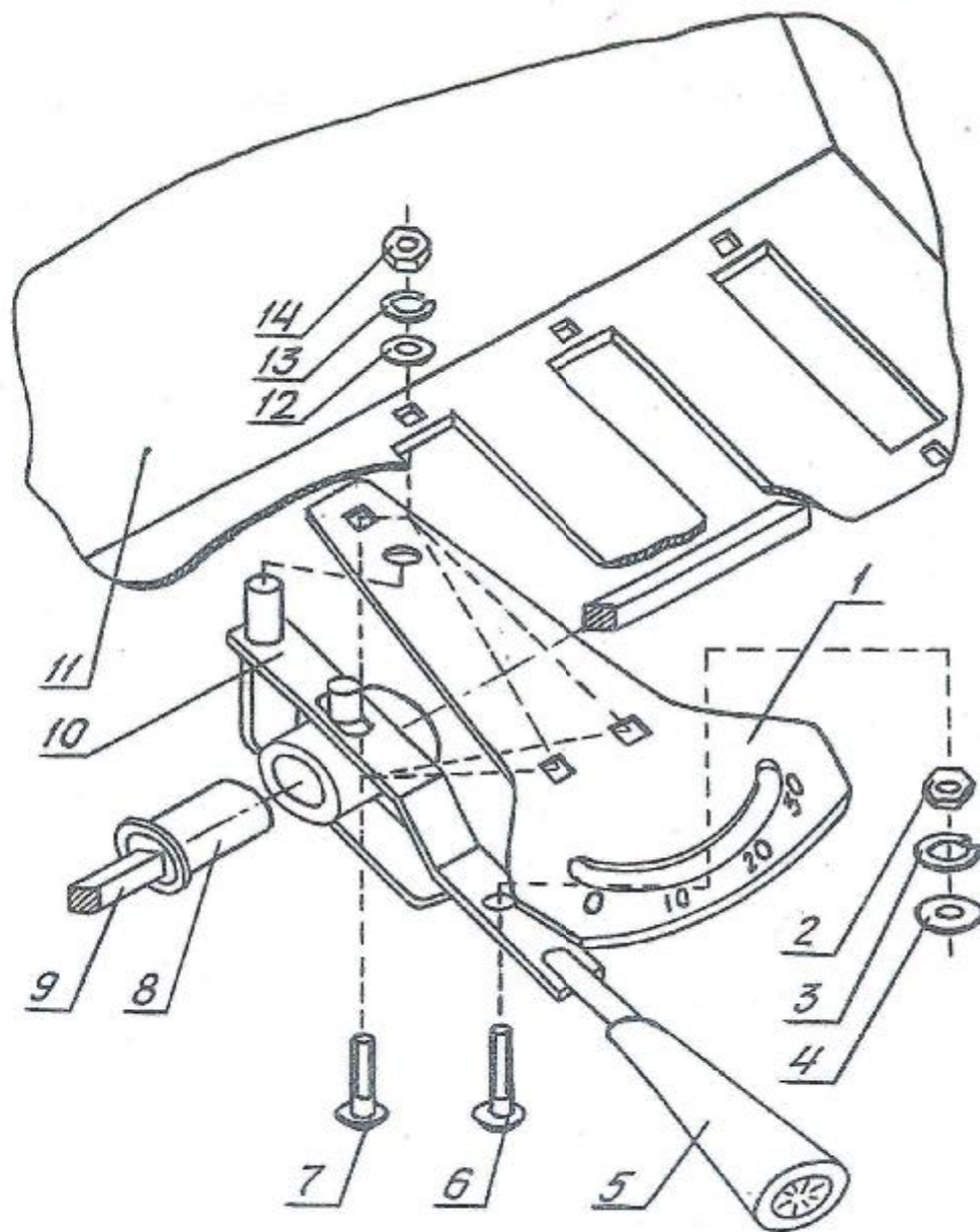
Рис. 17 Механизм регулировки нормы высева семян зерновых аппаратов
