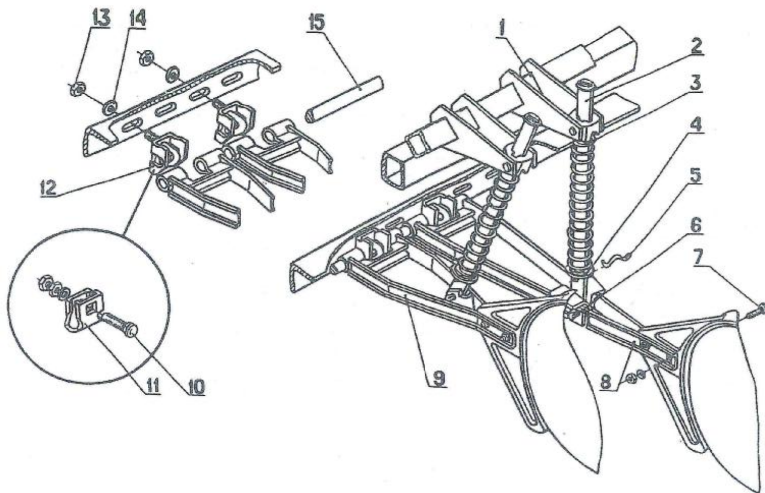
Рис. 9 Механизм навески сошников
