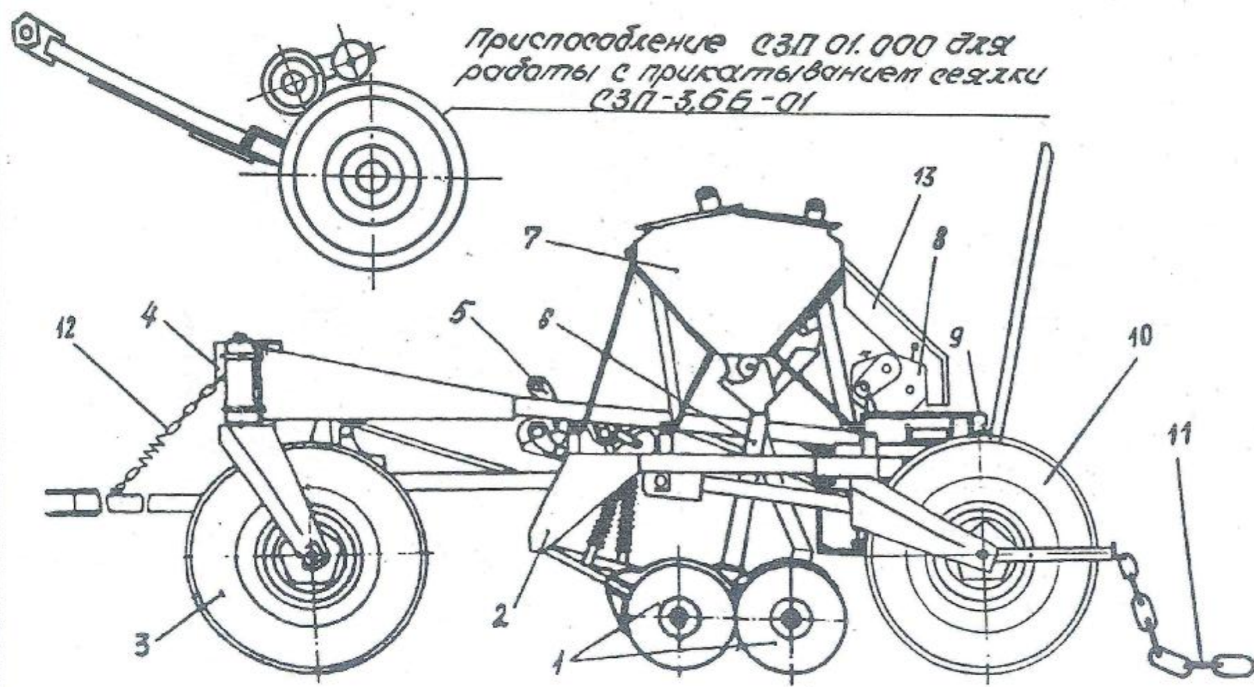
Рис. 3 Общее устройство сеялки СЗП-3,6Б-01
