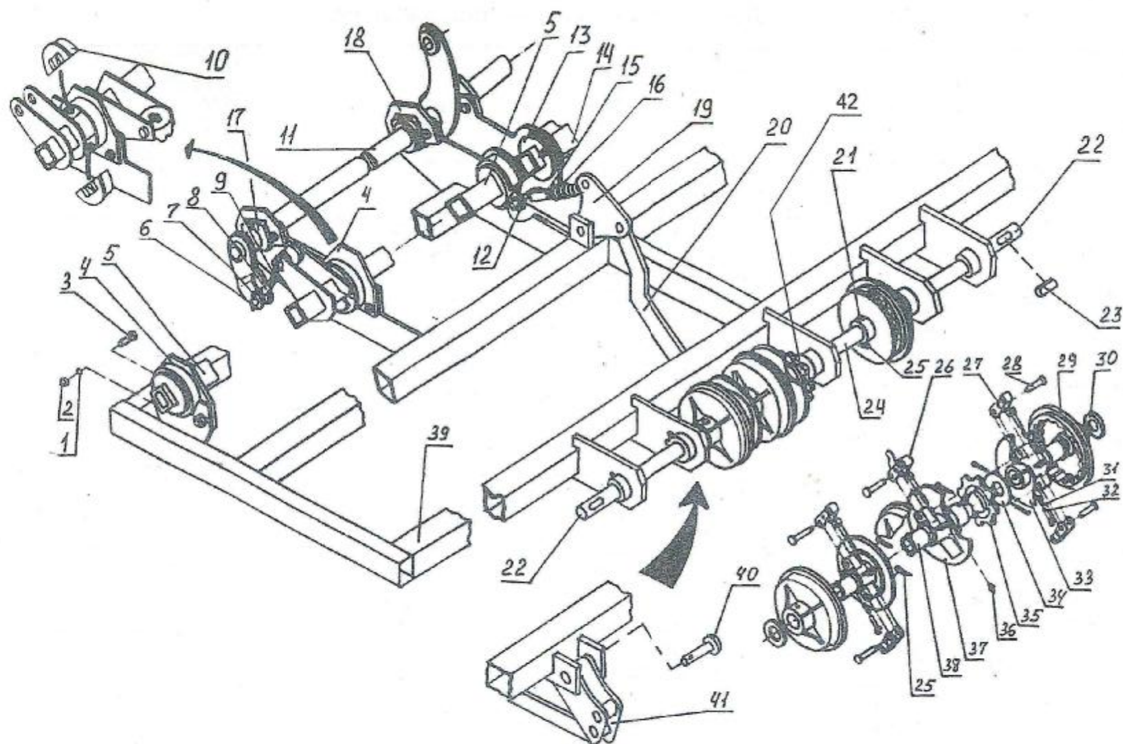
Рис. 6 Установка валов подъема сошников и механизма контрпривода
